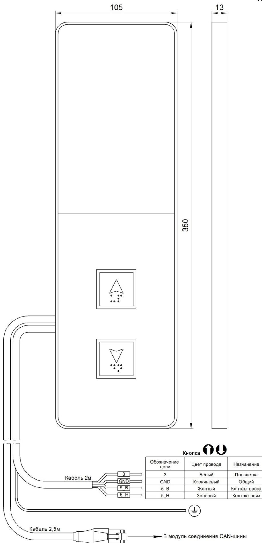
Рис.1 Внешний вид, габаритные и установочные размеры Вызывного поста МАЛАХИТ (жгут RJ45) НШЕК.468381.087
